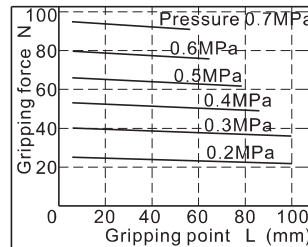
HFZ32\HFK32
